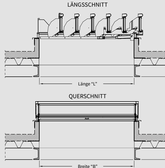
TECHNISCHE BEISPIELDATEN - ABMESSUNGEN (BREITEN u. LÄNGEN) UND DAZUGEHÖRIGE Av-WERTE (m 2 )
