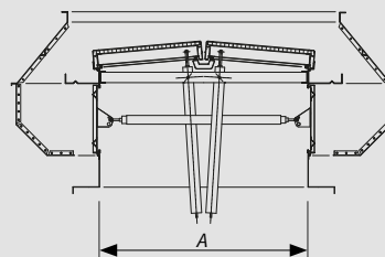
Basisausführung B2 (isolierte Ausführung)
